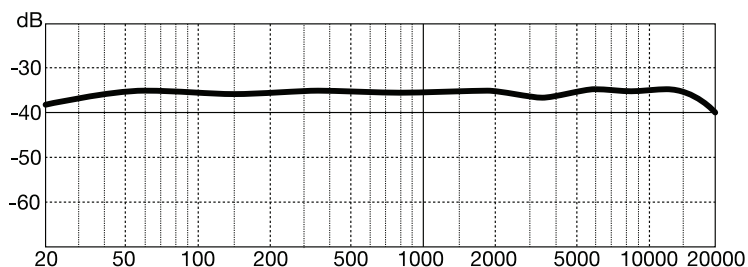
Частотный отклик
